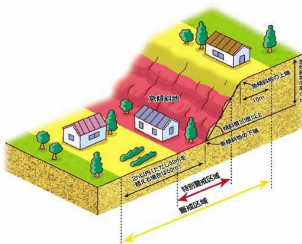
区域指定のイメージ(がけ崩れ)
